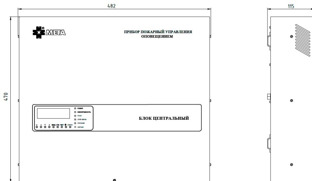
Рисунок 2. Габаритные размеры ЦБ МЕТА 17820/17821.
