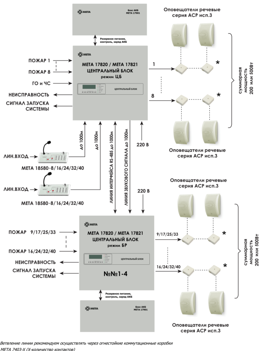
Рисунок 13. Структурная схема, построенная на базе ЦБ META 17820/17821.
