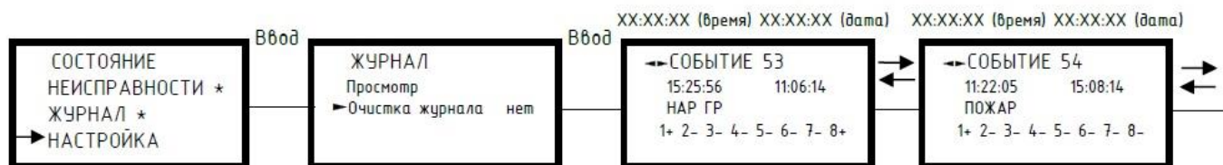
Рисунок 36. Журнал событий.
