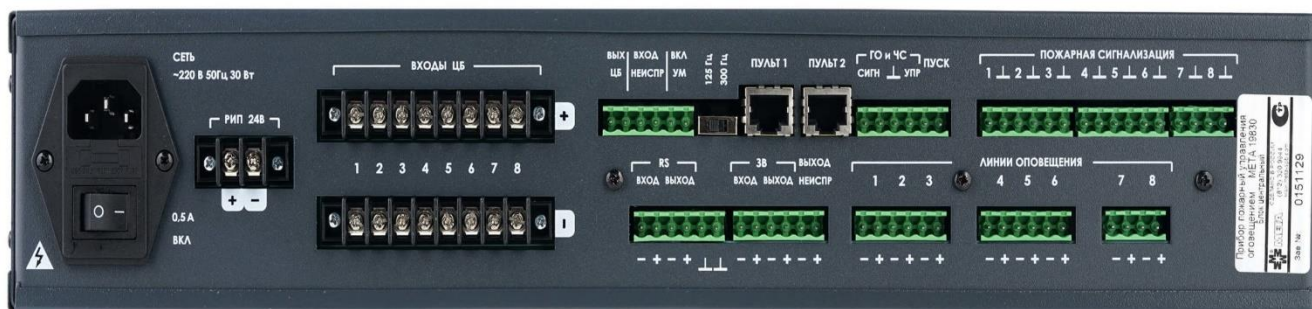
Рисунок 5. Задняя панель и расположение разъемов ЦБ МЕТА 19830.
