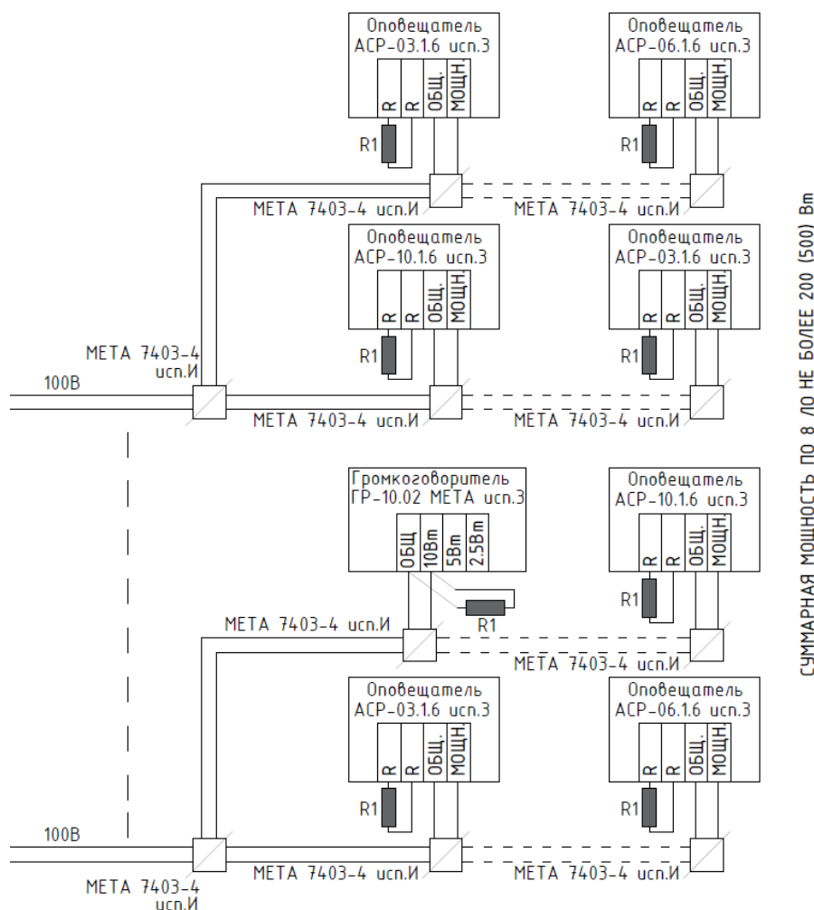
Рисунок 18. Схема подключения речевых оповещателей на ЛО.
