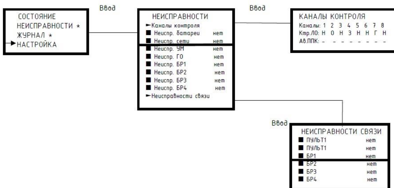
Рисунок 35. Окно НЕИСПРАВНОСТИ.
